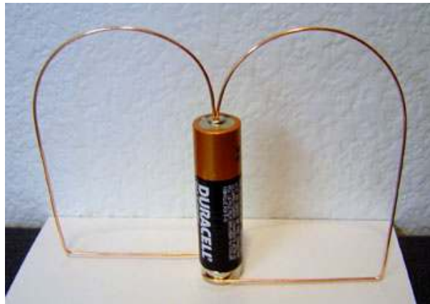
Moteur homopolaire
